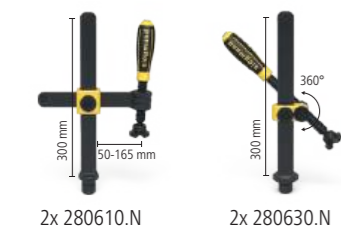
2x 280610.N
